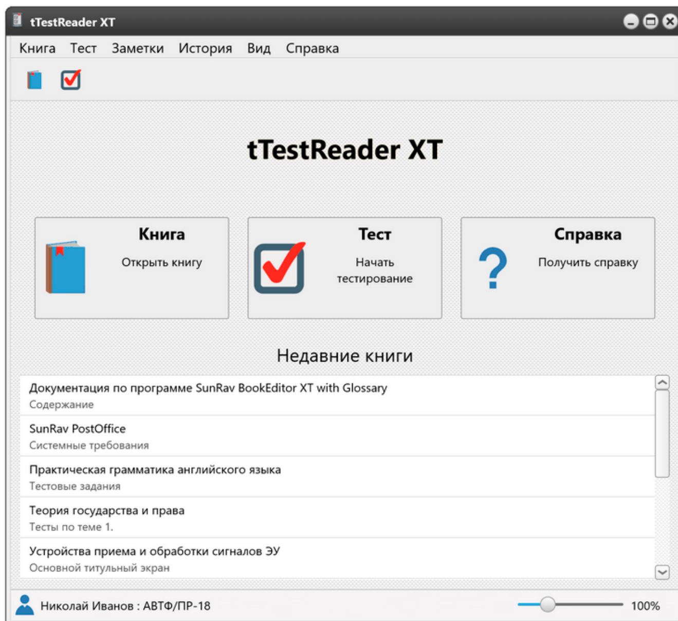
Рис. 3. Начальное окно программы
